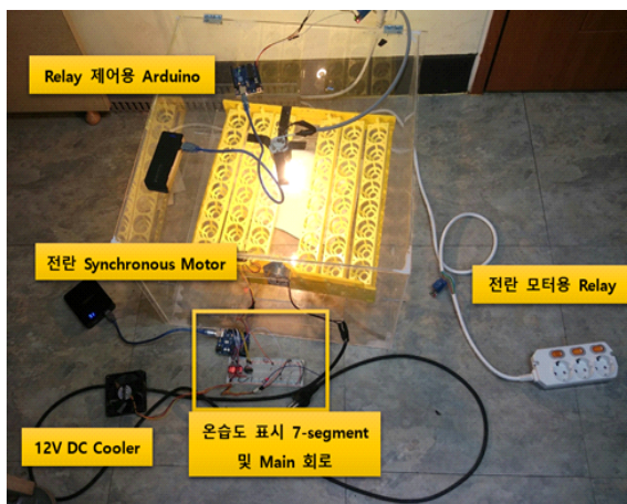
<ATET에서 아이템을 발굴하여 제작한 병아리 부화기 장비>
